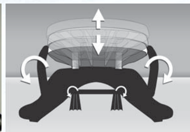
beidseitig wirkende Bremse | static brake
